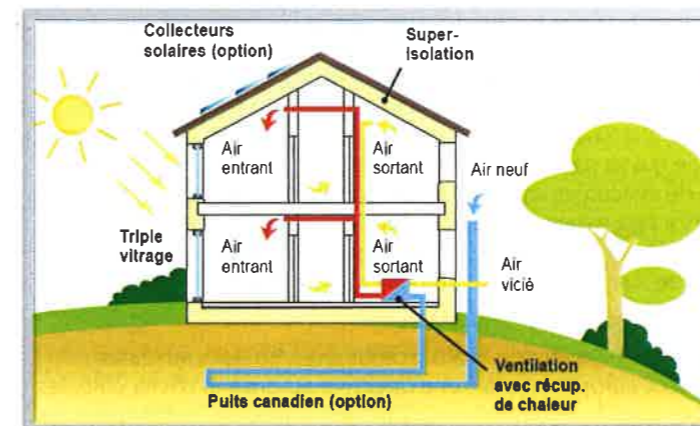
Schéma de principe d'une maison passive – FFCP
